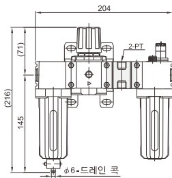
PACT300L-T* T-타입 마운트 브래킷
