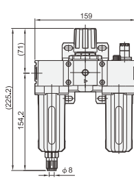
PACT300L-D (오토 드레인) 압력설정범위 : 0.15~0.99MPa
